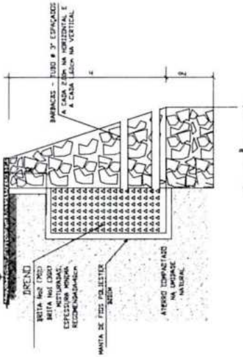
CORTE - MURO DE CONTENÇÃO SEM ESC.
