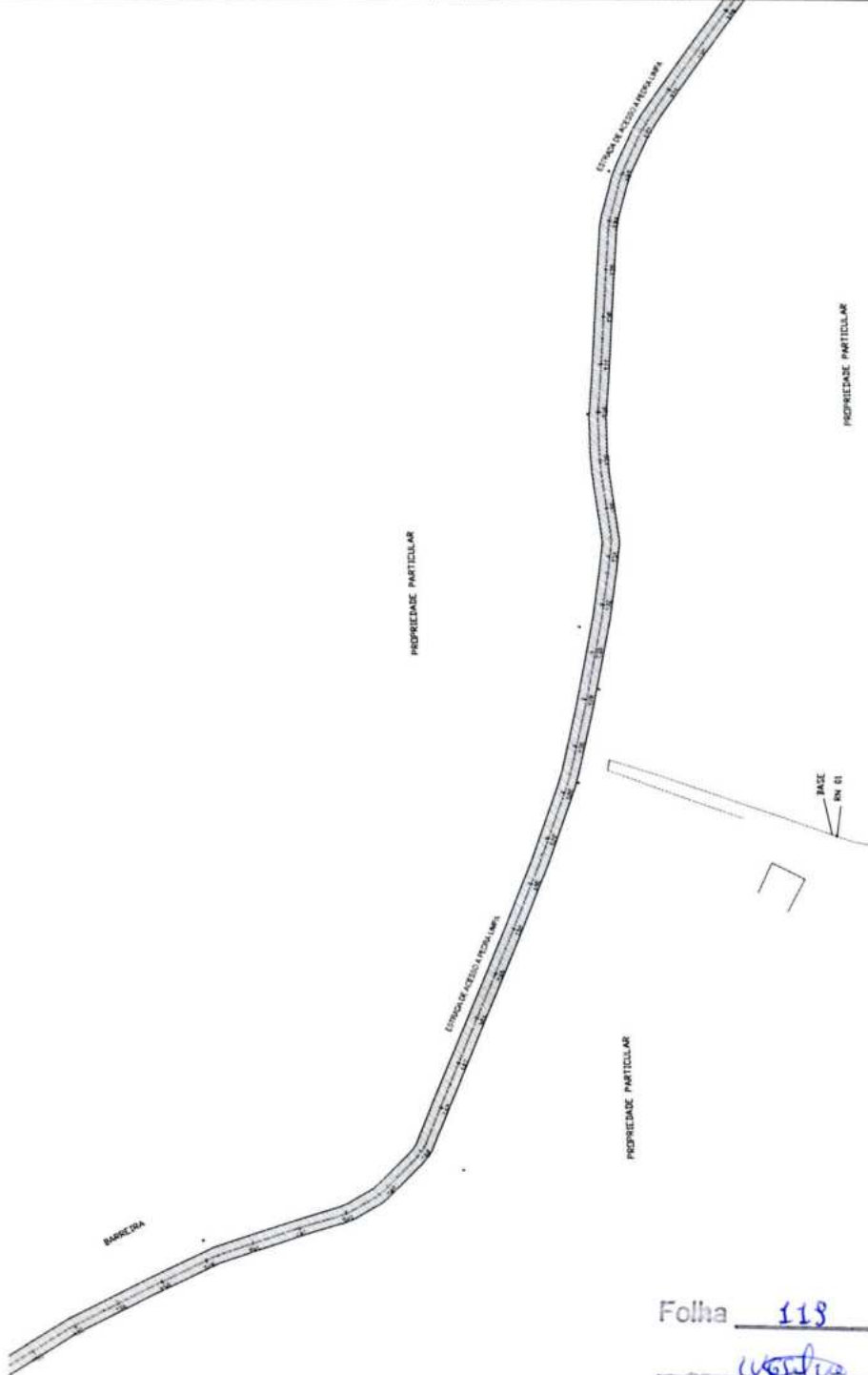
PLANTA PAVIMENTAÇÃO - TRECHO 02 E.C. 1/100
