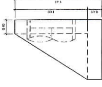
VISTA (PONTA DE ALA) SESCALA
