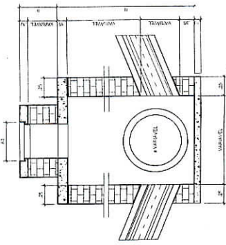
CORTE A-A (POÇO DE VISITA) SESCALA
